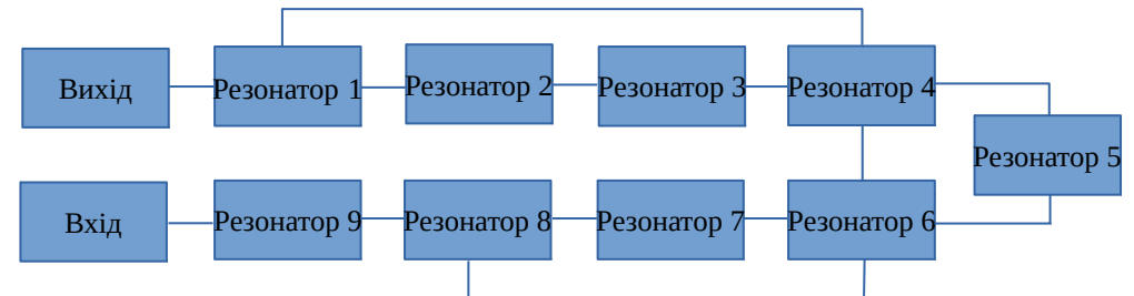
Структурна схема радіочастотного смугового фільтра “ФС-820-2-30”
