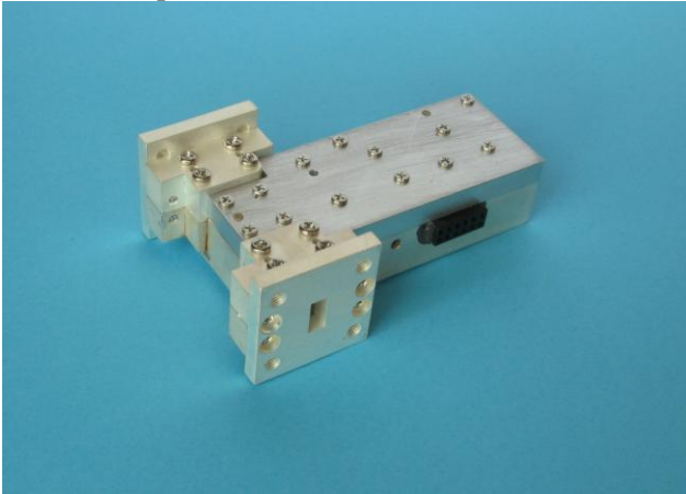
Рис. 6. Умножительно-разветвительный модуль
