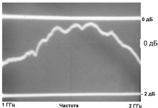
Рис. 12. Проходная частотная характеристика приемно-передающего тракта
