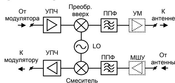
Рис. 1. Структурная схема приемно-передатчика
