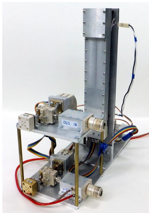
Рис. 11. Приемо-передатчик для радиорелейной системы терагерцового диапазона
