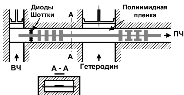
Рис. 2. Конструкция преобразователя
