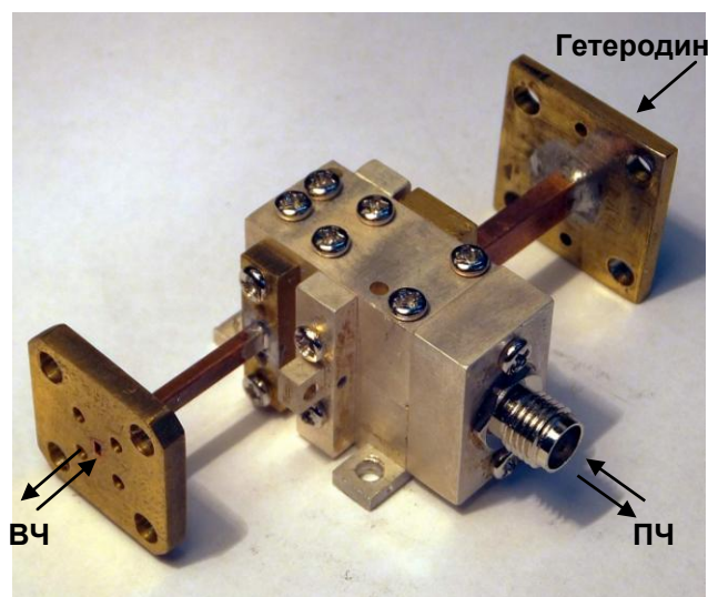
Рис. 3. Частотный преобразователь с присоединенными отрезками волноводов
