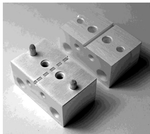
Рис. 9. Фотография septum-фильтра (в разобранном виде)
