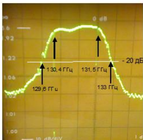
Рис. 10. Измеренная АЧХ фильтра
