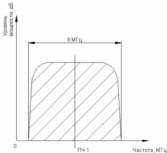
Рис. 2. Спектр сигнала на выходе модулятора M-QAM
