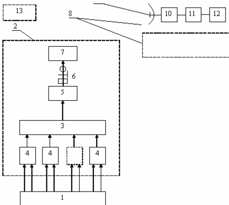
Рис. 1. Структурная схема микроволновой интегрированной телерадиоинформационной системы МИТРИС–МЮИ: 1 – Подсистема приема, формирования и обработки информации; 2 – Центральная станция; 3 – Программируемый конвертер –формирователь группового сигнала промежуточной частоты; 4 – Комбинированный модулятор M-QAM/FM; 5 – СВЧ передатчик; 6 – Соединительная радиочастотная линия; 7 – Антенное устройство; 8 – Абонентская приемная станция; 9 – Антенна абонентской станции; 10 – Малошумящий конвертер; 11 – Селективный демодулятор– преобразователь частоты; 12 – Демодулятор стандарта DVB–С; 13 – Ретранслятор
