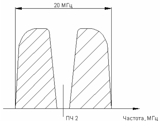
Рис. 3. Спектр сигнала на выходе модулятора FM.
